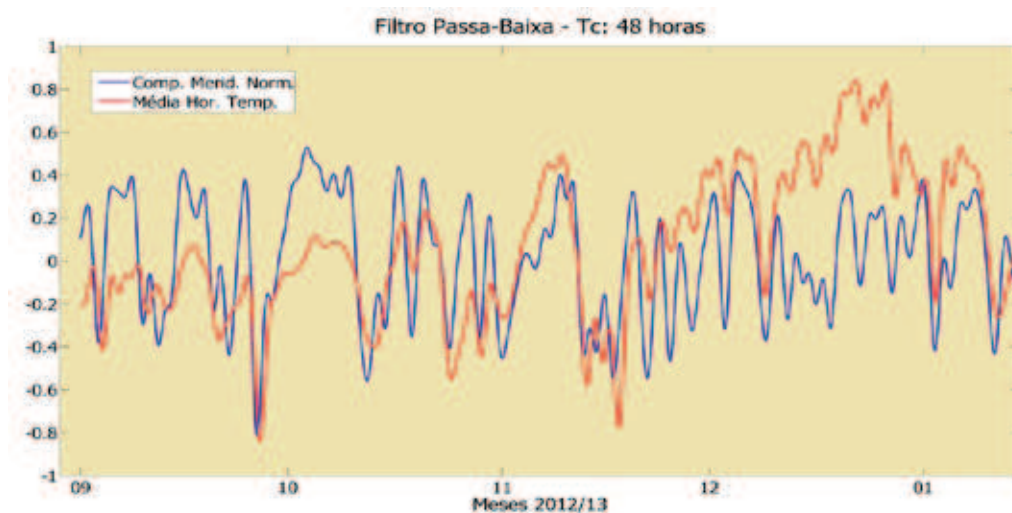
Figura 4 - Comparação entre a média horária da temperatura na Enseada dos Anjos com a componente meridional (norte-sul) do vento, ambas normalizadas e submetidas a uma filtragem passa-baixa ( T_c = 48 h), destacando-se a estreita relação entre o comportamento das duas séries.
