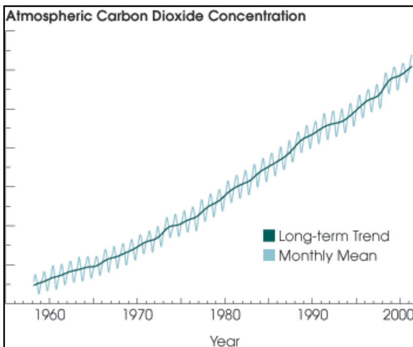
FIGURA 7 – Concentração de dióxido de carbono na atmosfera - 1958 a 2001.
