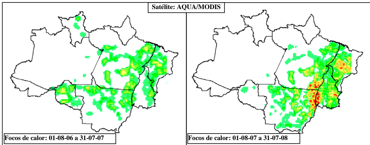
FIGURA 8 – Queimadas na Amazônia Legal, de 2006 a 2008 (as tonalidades verde, amarelo e vermelho representam o aumento no número de focos por célula).
